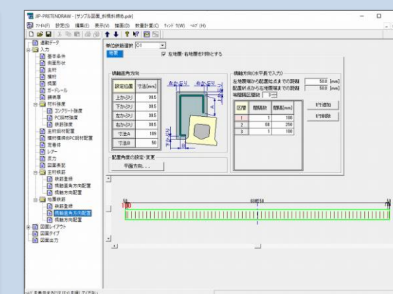
入力/地覆鉄筋 - 橋軸直角方向配置
